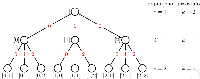
Slika 5.4: Postupak generisanja varijacija sa ponavljanjem dužine k = 2 , za n = 3 .
